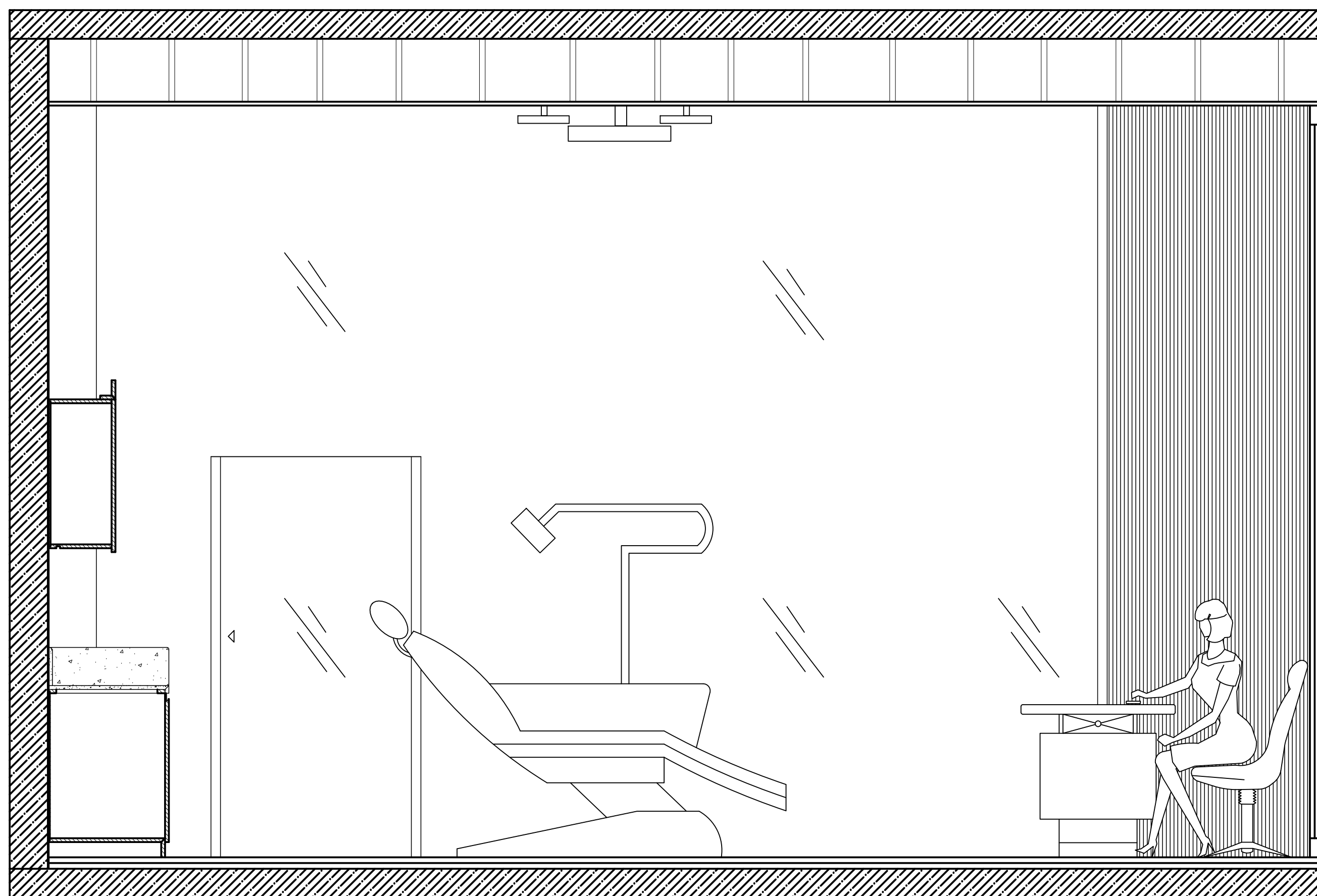
D-D KESİTİ:
