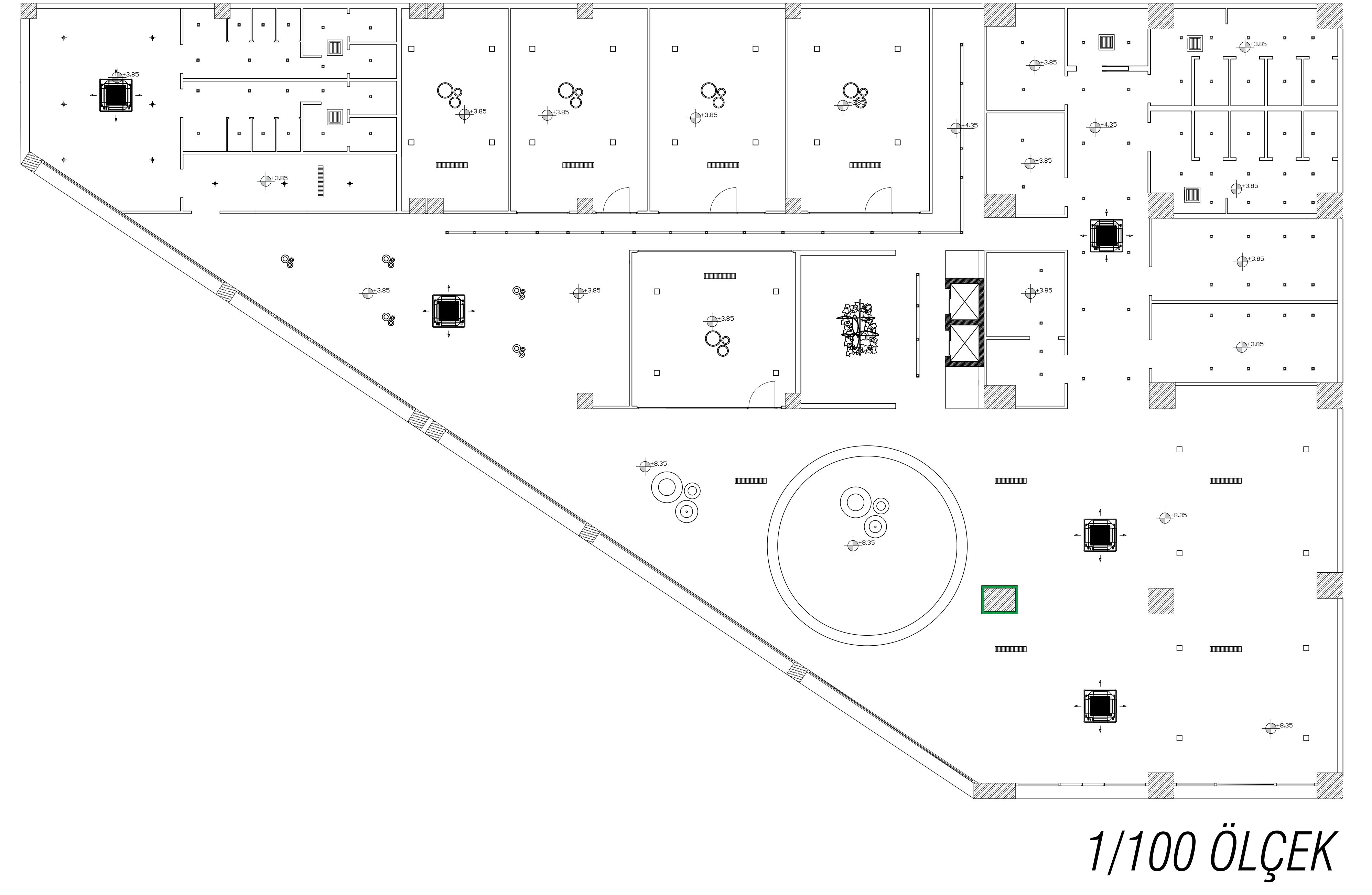
ZEMİN KAT TAVAN PLANI:
